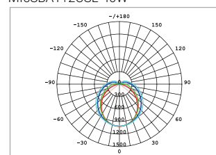
MI5SBA112CSL-40W
